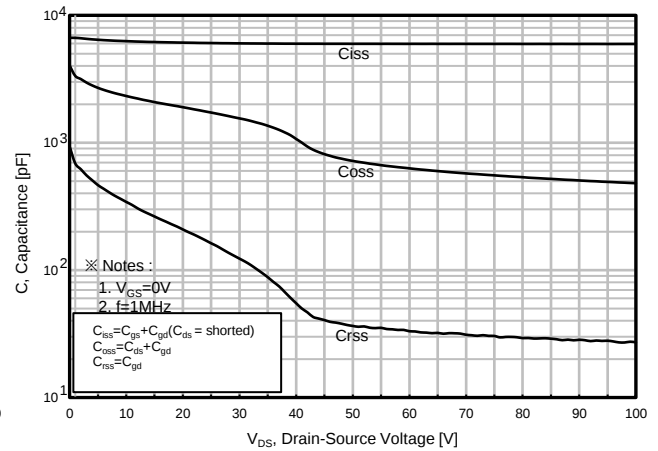
Fig. 8. Capacitances
