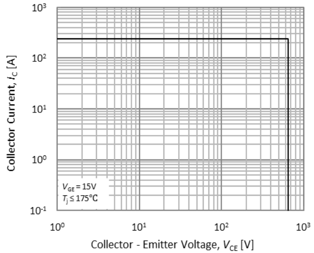
Fig.28. RBSOA
