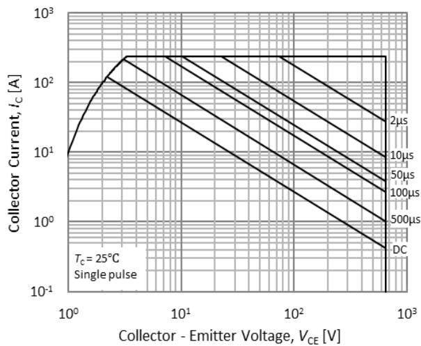
Fig.27. FBSOA
