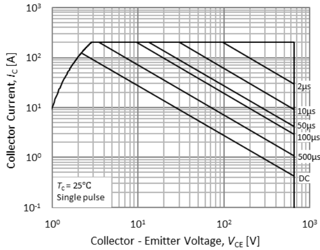
Fig.27. FBSOA
