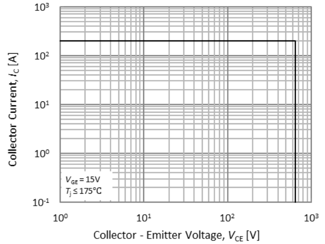
Fig.28. RBSOA
