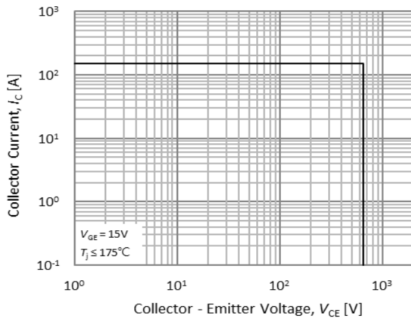
Fig.25. RBSOA
