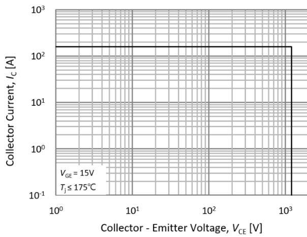
Fig.25. RBSOA
