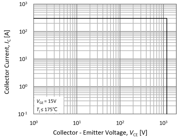
Fig.28. RBSOA
