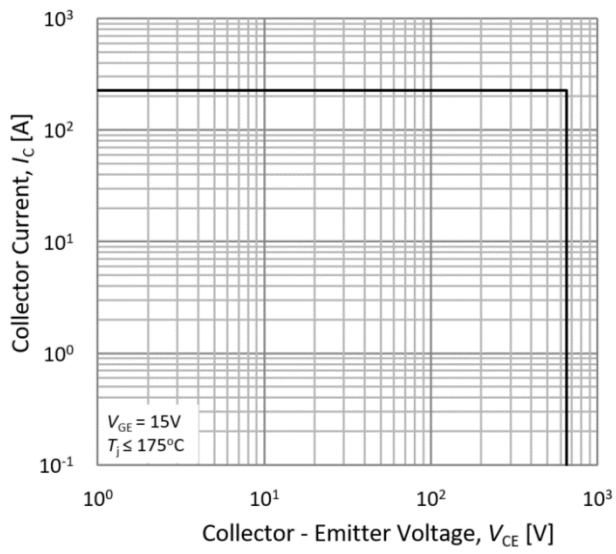
Fig.22. RBSOA
