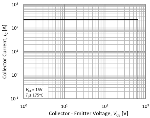
Fig.23. RBSOA
