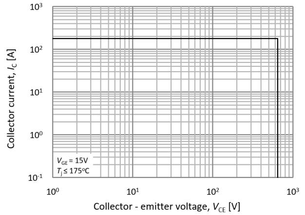
Fig.22 RBSOA
