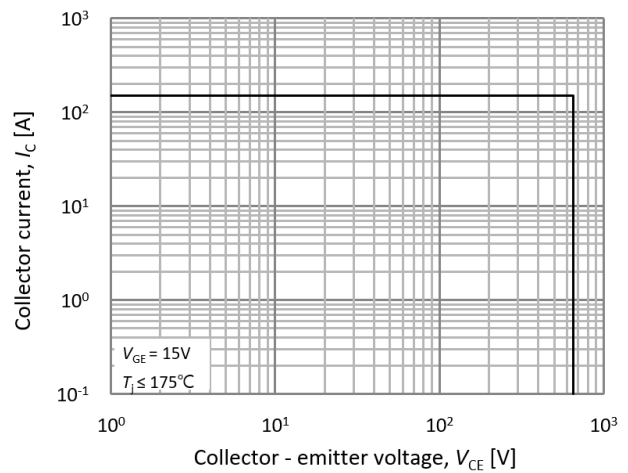
Fig.22. RBSOA
