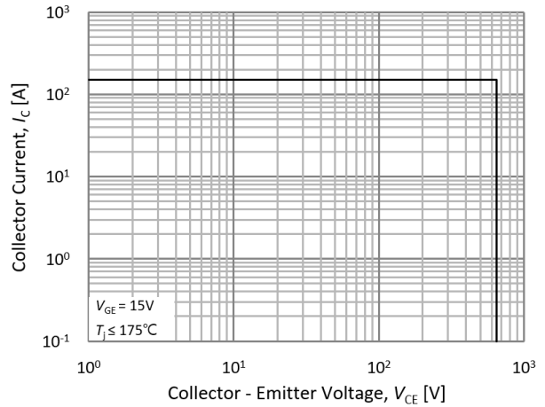
Fig.22. RBSOA
