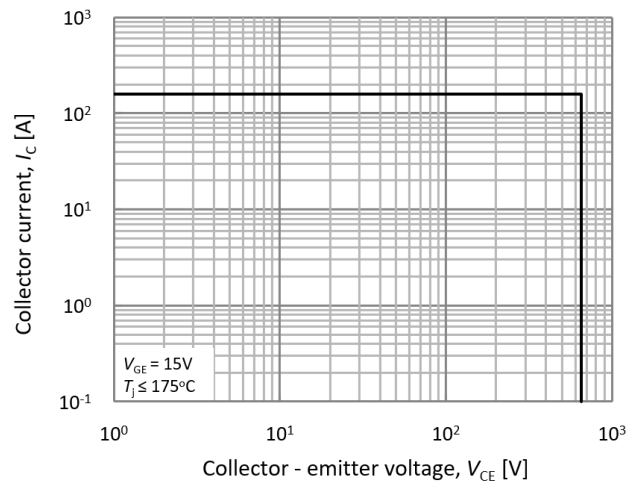
Fig.22. RBSOA
