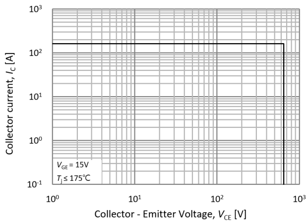
Fig.25. RBSOA
