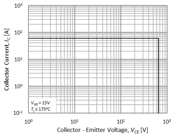
Fig.23. RBSOA
