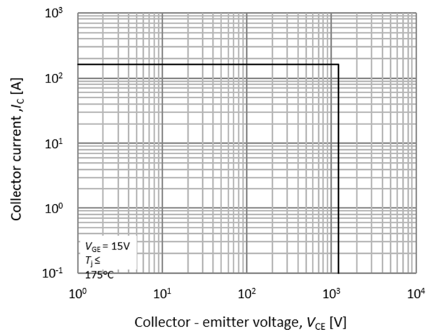
Fig.18 RBSOA
