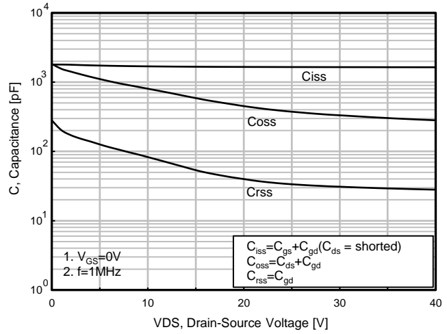
Fig. 8. Typ. Capacitances
