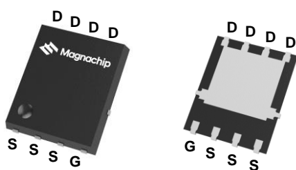
PowerDFN56
