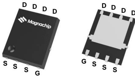
PowerDFN56
