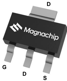
SOT-223
