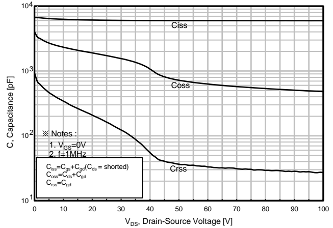
Fig. 8. Capacitances
